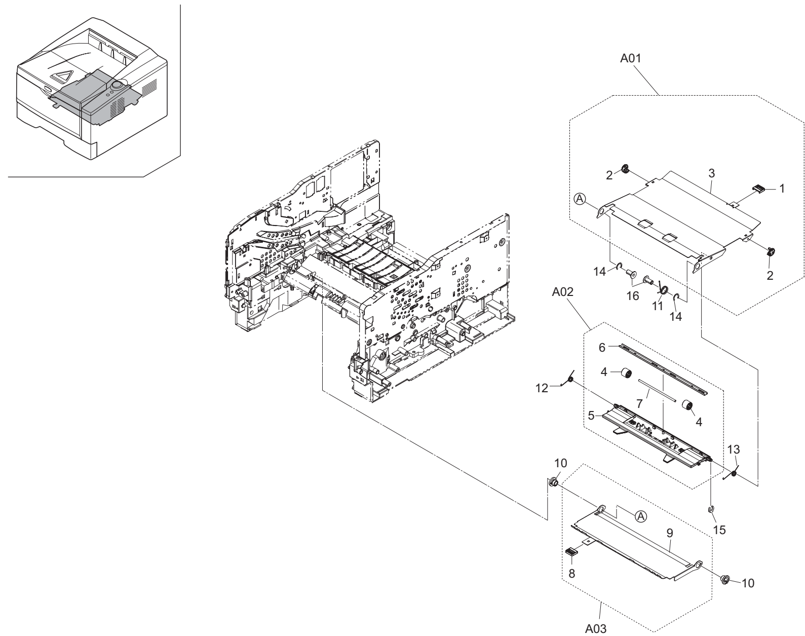
FIG. 10 Duplex Section
